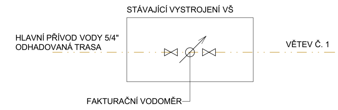
SCHÉMA "A"
