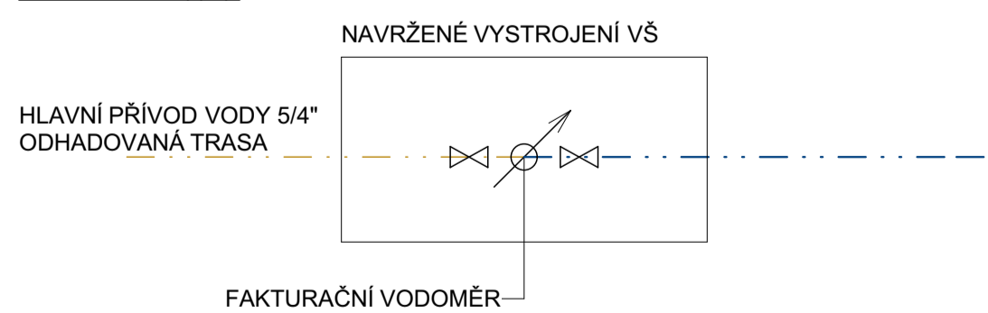
SCHÉMA "B"
