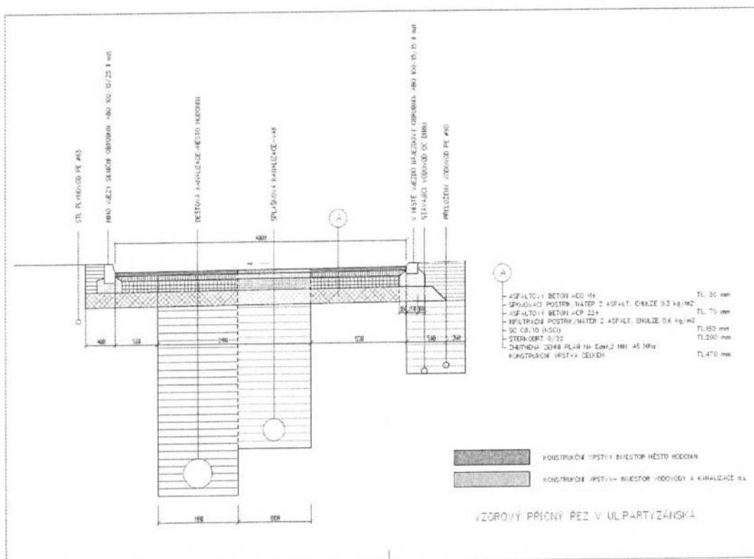
Obr. č.2: Aktualizovaný vzorový řez
