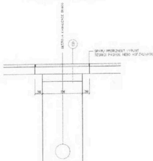
ZAPRAVENÍ RÝHY V KOMUNIKACI PODKLADNÍ VRSTVA Z BETONU
