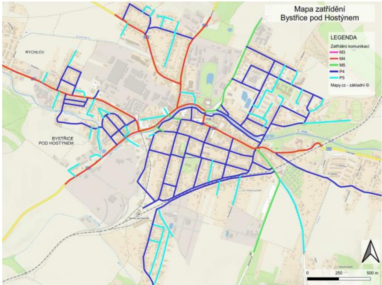
Zatřídění komunikací dle ČSN CEN/TR 13201-1
