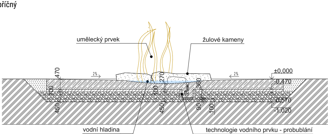
D1 řez příčný
