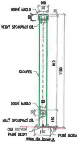
ŘEZ B-B'
