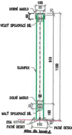
ŘEZ B-B'
