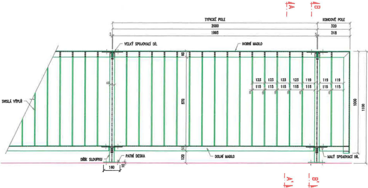
POHLED NA ZÁBRADLÍ 1:10
