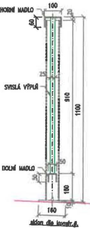
PŘÍČNÉ ŘEZY 1:10 ŘEZ A-A'
