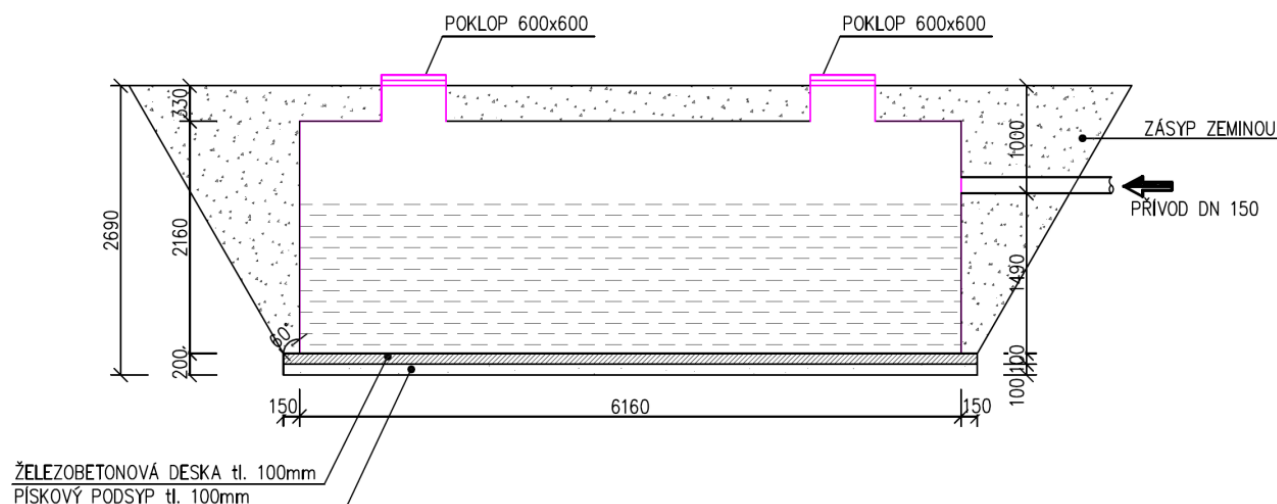
VÝKRES Č. 204 - SO 02 - BEZODTOKOVÁ JÍMKA - ULOŽENÍ
