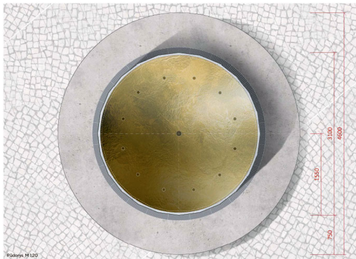
Přehled M 1:20
