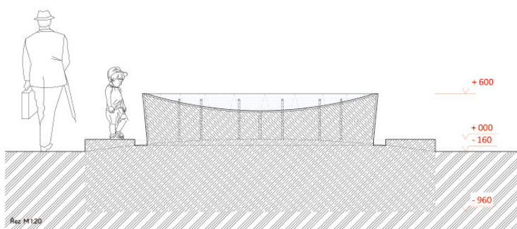
Ráz M 1:20
