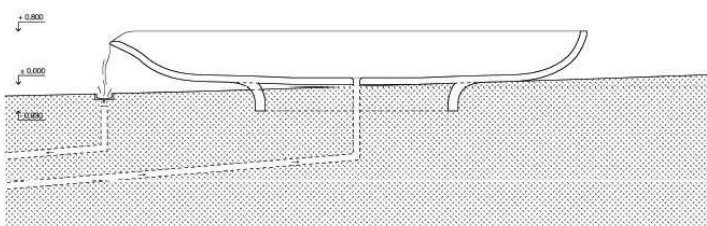
řez
